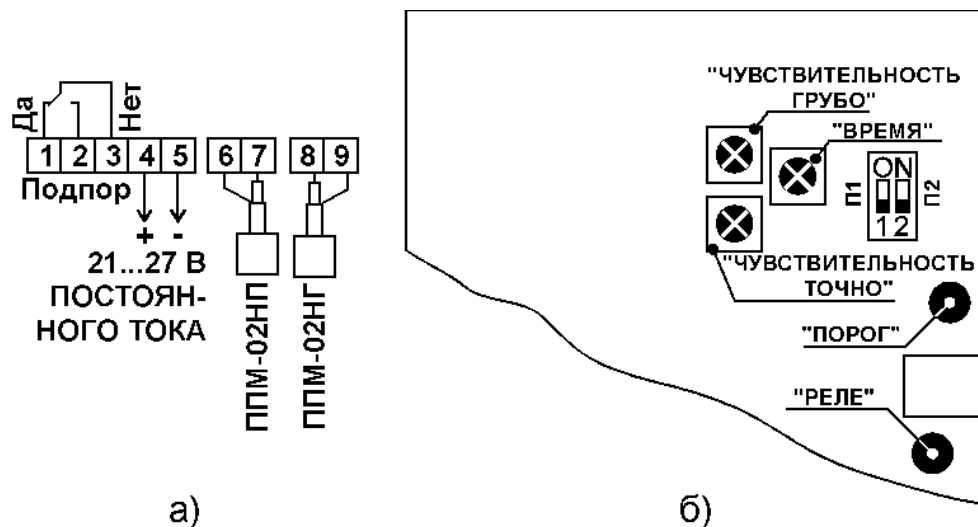
Рис. 5. Схема подключения и органы регулировки датчика.
